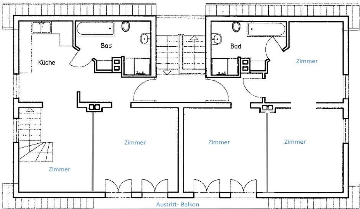
untere Ebene
