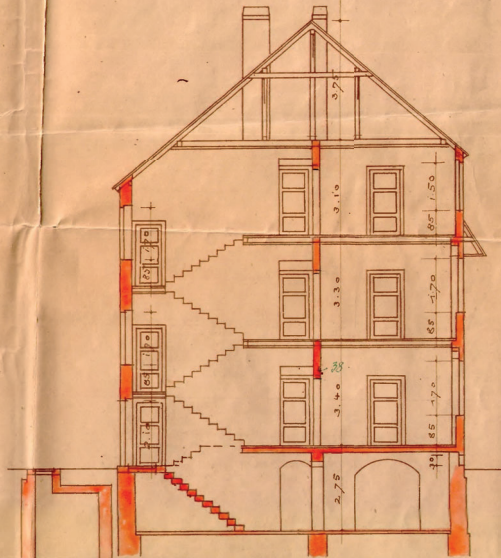
QUERSCHNITT
