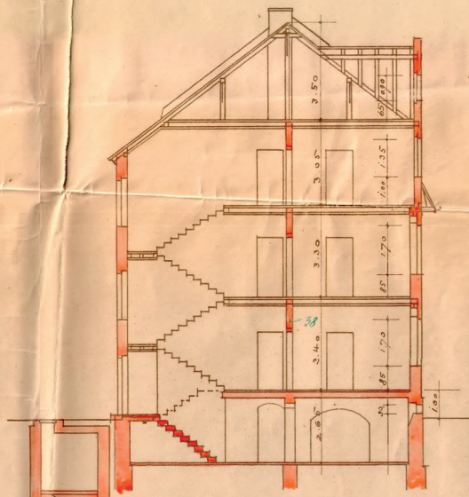
QUERSCHNITT. basile & Flachsmaier.
