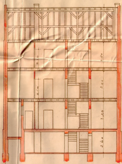
LÄNGENSCHNITT.
