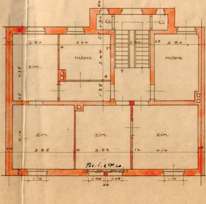
I. OBERGESCHOSS.
