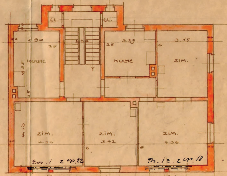
I. OBERGESHOSS.
