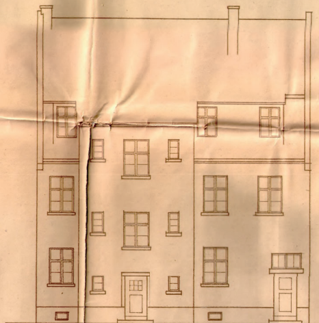
RÜCKANSICHT.
