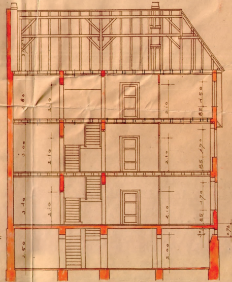
LANGENSCHNITT.
